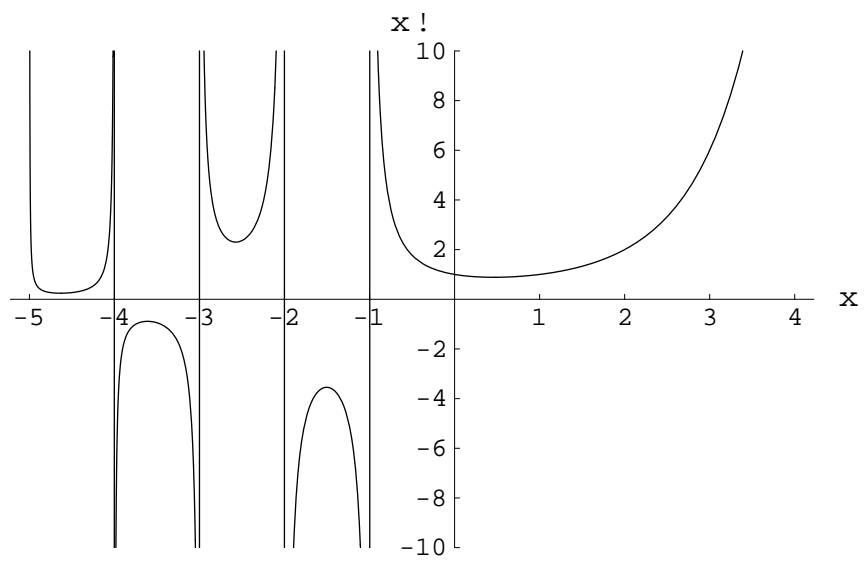
Abbildung 5.1: Die reelle Fakultätsfunktion x! = \int_0^\infty t^x e^{-t} dt .
